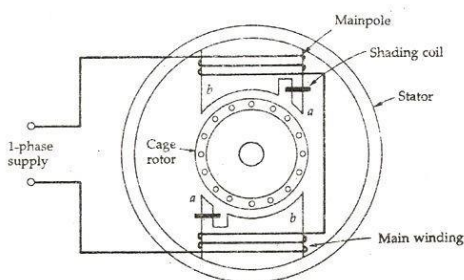
รูปที่ 6 แผนผังแสดงการต่อขดลวดของมอเตอร์ไฟฟ้ากระแสสลับเหนี่ยวนำเฟสเดียว แบบ Shaded pole motor 9
