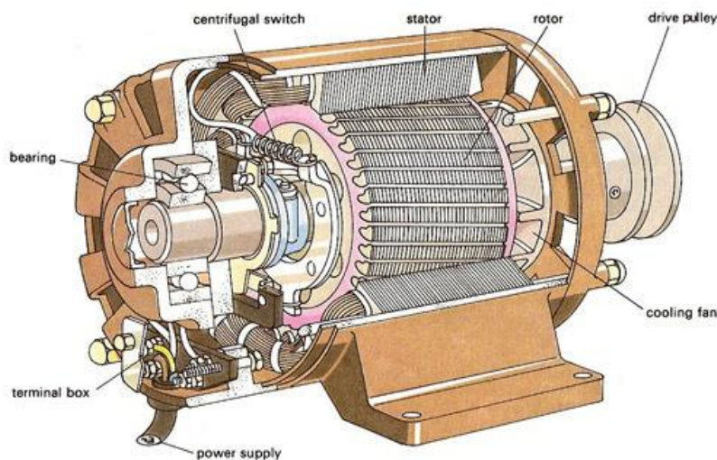
รูปที่ 1 ภาพตัดขวางของมอเตอร์ไฟฟ้ากระแสสลับเหนี่ยวนำแสดงส่วนประกอบต่าง ๆ ภายใน 3
