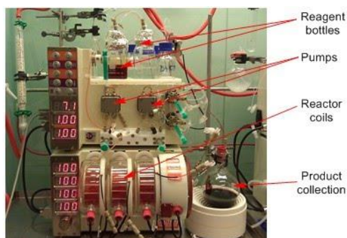
รูปที่ 1 แสดงอุปกรณ์ของเคมีการไหล ที่มา: Dr Wallace W. H. Wong (2014)
