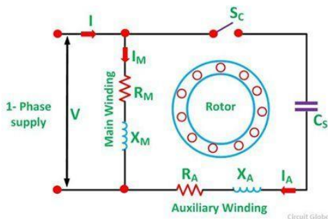
รูปที่ 3 แผนผังแสดงการต่อขดลวดของมอเตอร์ไฟฟ้ากระแสสลับเหนี่ยวนำเฟสเดียว แบบคาปาซิเตอร์สตาร์ทมอเตอร์ 5
