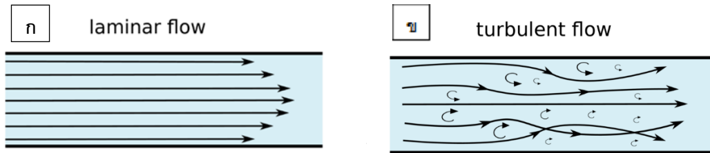
รูปที่ 10 แสดงลักษณะการไหล (ก) แบบสม่ำเสมอและ (ข) การไหลแบบปั่นป่วน ที่มา: CFDsupport (2018)
