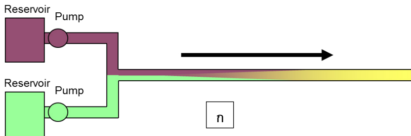
รูปที่ 11 แสดงตำแหน่งของระยะทางที่สัมพันธ์กับเวลาที่เกิดการแพร่สมบูรณในรีแอกเตอร์ ที่มา: Plutschack MB et al. (2017)
