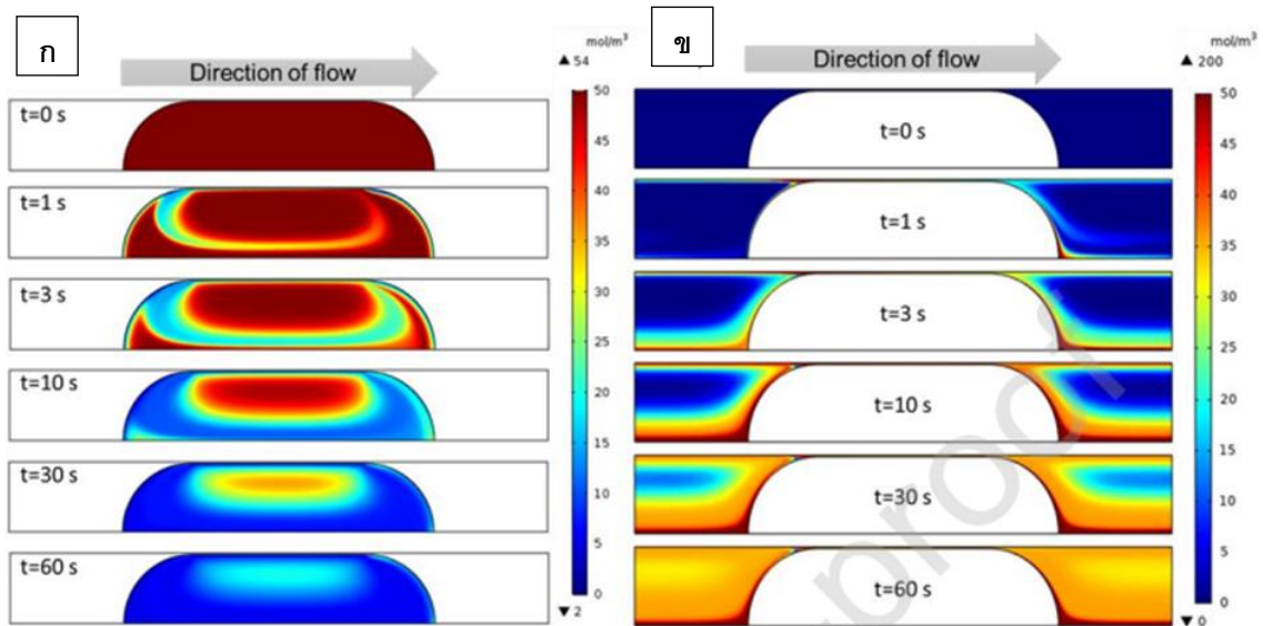
รูปที่ 9 แสดงลักษณะการถ่ายโอนของเฟสภายใน (ก) และเฟสภายนอก (ข) ที่ระยะต่าง ๆ ในรีแอกเตอร์ ที่มา: Eduardo Garciadiego-Ortega et al. (2020)
