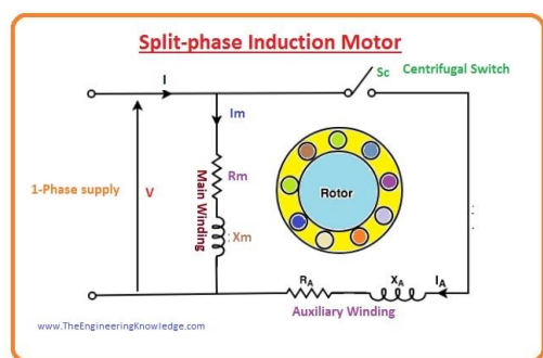
รูปที่ 2 แผนผังแสดงการต่อขดลวดของมอเตอร์ไฟฟ้ากระแสสลับเหนี่ยวนำเฟสเดียว แบบสปลิตเฟส 4
