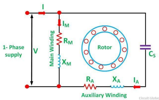
รูปที่ 5 แผนผังแสดงการต่อขดลวดของมอเตอร์ไฟฟ้ากระแสสลับเหนี่ยวนำเฟสเดียว แบบมอเตอร์ชนิดที่มีคาปาซิเตอร์ถาวร 8
