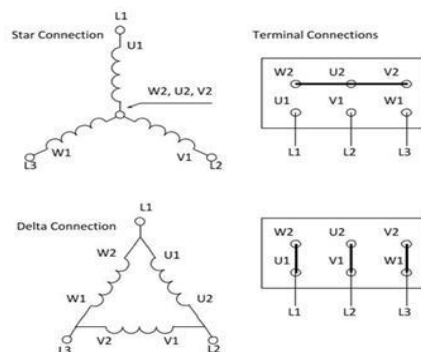
รูปที่ 8 แผนภาพแสดงการต่อวงจรแบบสตาร์ทและแบบ เดลต้าของมอเตอร์ไฟฟ้ากระแสสลับเหนี่ยวนำสามเฟส 12
