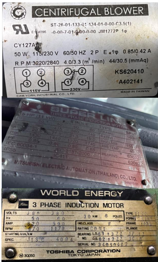
รูปที่ 9 ตัวอย่างแผ่นป้ายชื่อของมอเตอร์ไฟฟ้า กระแสสลับเหนี่ยวนำสามเฟสแบบ 2, 4 และ 6 ขั้วเรียงจากบนลงล่าง (ภาพของผู้นิพนธ์)
