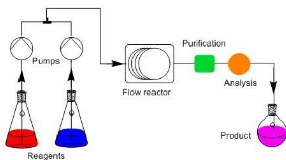
รูปที่ 1 แสดงอุปกรณ์ของเคมีการไหล ที่มา: Dr Wallace W. H. Wong (2014)
