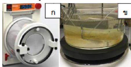
รูปที่ 8 แสดงลักษณะของอุปกรณ์ควบคุมความร้อนแบบ (ก) ฮีทแจ็คเก็ตและแบบ (ข) อ่างน้ำร้อน
