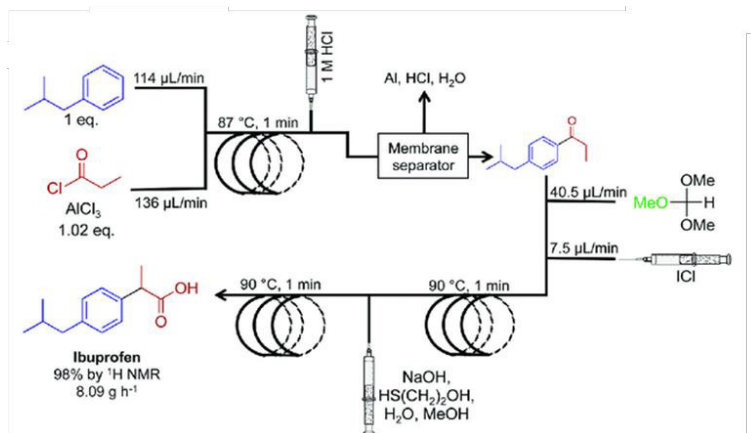
รูปที่ 15 แสดงระบบเคมีไหลในการสังเคราะห์ไอบูโพรเฟนของเจมิสัน (Jamison) และคณะ ที่มา: Britton J, Jamison TF (2017)
