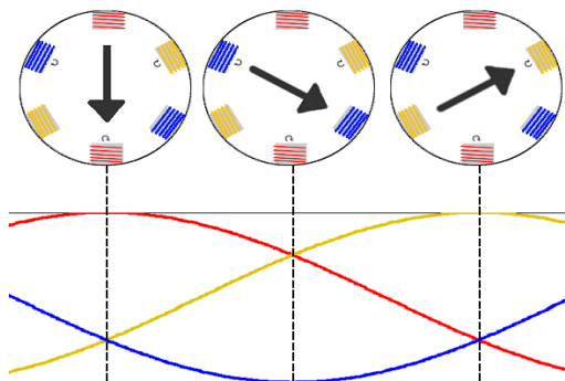
รูปที่ 7 แผนภาพแสดงการทำงานของมอเตอร์สามเฟส 11
