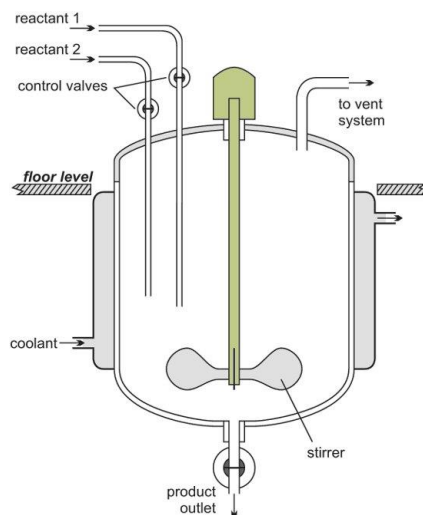
รูปที่ 1 แสดงอุปกรณ์สังเคราะห์สารในถังผสม ที่มา: The Essential Chemical Industry – online (2013)
