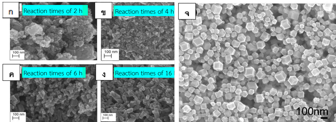
รูปที่ 16 แสดงลักษณะผลิตภัณฑ์การสังเคราะห์อนุภาคไขมันแข็งของซีโอไลติก-อิมิดาโซลเลตที่สังเคราะห์ด้วยการผสมในถังผสมที่เวลา (ก) 2 ชั่วโมง (ข) 4 ชั่วโมง (ค) 6 ชั่วโมง (ง) 16 ชั่วโมงและ (จ) ผลิตภัณฑ์ที่ได้จากเคมีกรไล
